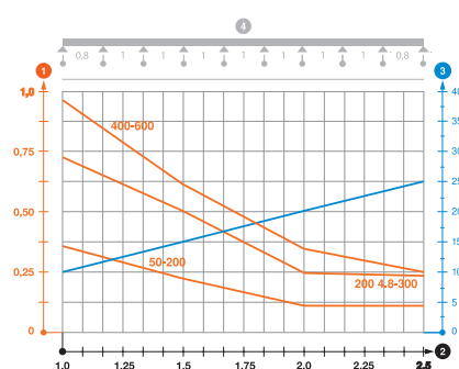
Belastningsdiagram C-gitterbakke GRM 55 VA
